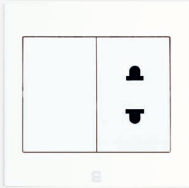
16A socket euro-american type with blank 7x7 Code: MDN-212-1 16A فيش (بريزة) طراز أمريكي بالحماية 16 امبير 7x7 بجانب سدة - مفرد
