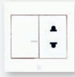
16A socket euro-american type + one way switch 7x7 Code: MDN-213-1 16A فیش (بریزة) طراز امريكي + مفتاح إضاءة 16 امبير 7x7 - مفرد
