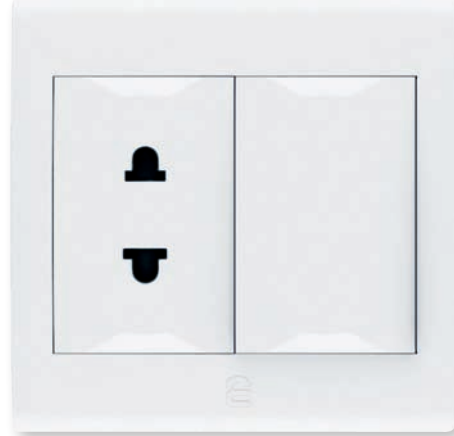
16A socket euro-american type with blank 7x7 Code: 707-212-1 16A فیش (بریزة) طراز أمريكي بالحماية 16 أمبير 7x7 – مفرد + سدة
