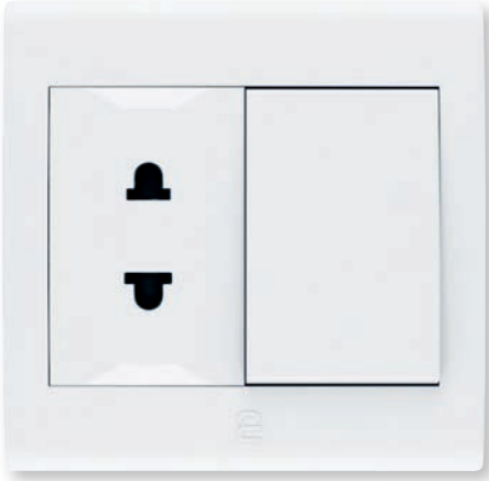
16A socket euro-american type with switch 7x7 Code: 707-213-1 16A فیش (بریزة) طراز أمريكي + مفتاح إضاءة 16 أمبير 7x7 – مفرد
